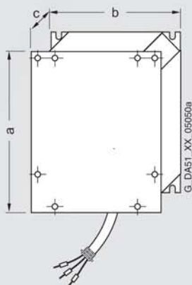
适合 B 型和 C 型外形尺寸 变频器的输出电抗器
