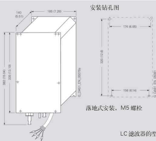
C 型变频器适用的 LC 滤波器
