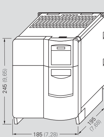
C 型外形尺寸的变频器
