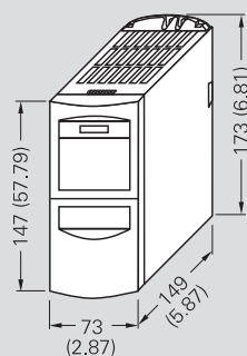
A 型箱体尺寸变频器
