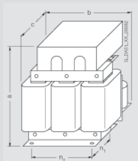
D 至 F 型变频器适用的 LC 滤波器
