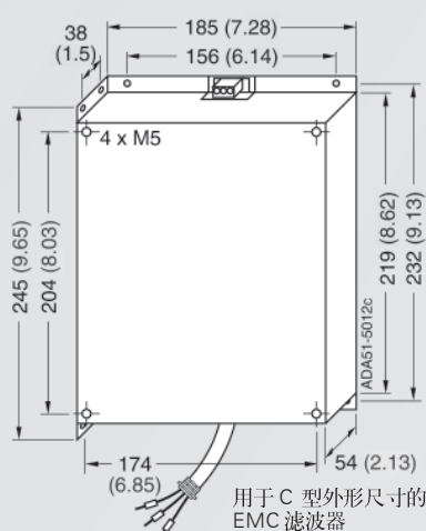
6SL3000- 型 A 级 EMC 滤波器
