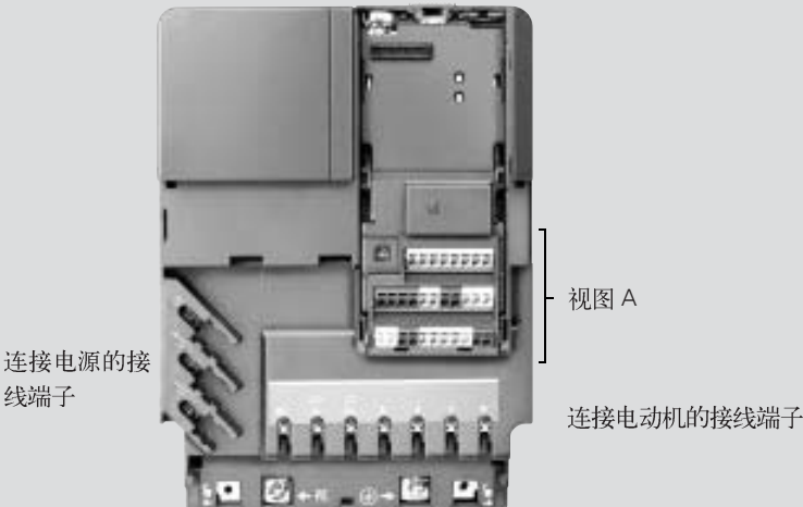
视图 A
