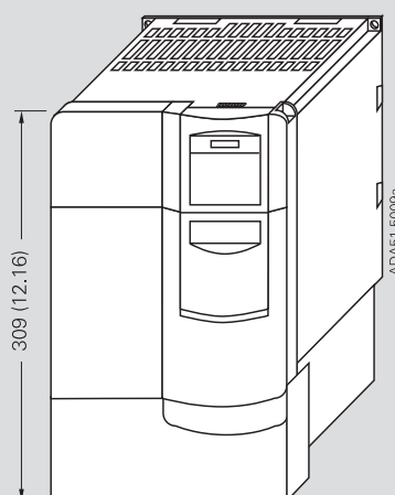
带有密封盖的 C 型箱体尺寸变频器 所有尺寸的单位都是 mm (括号内尺寸的单位是：英寸)
