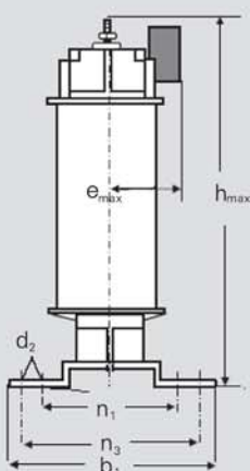
适合 A 型箱体国产进线电抗器
